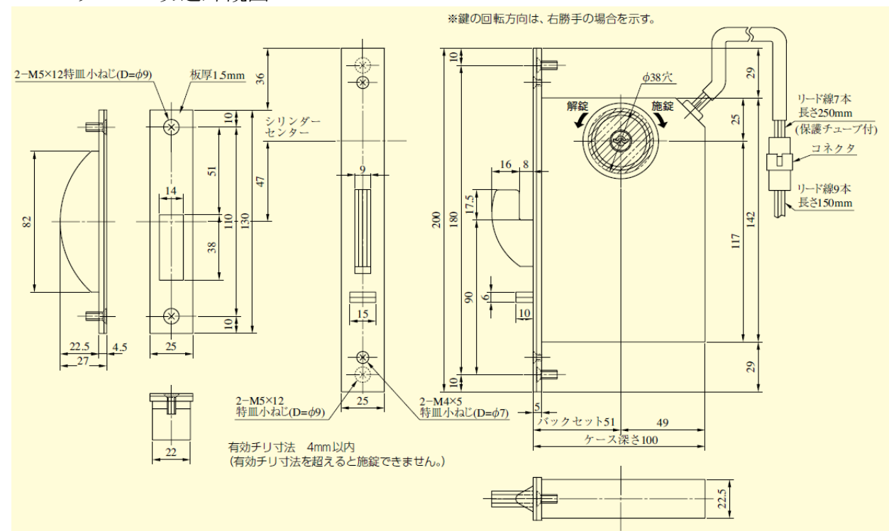
AFFシリーズの切込外観図
