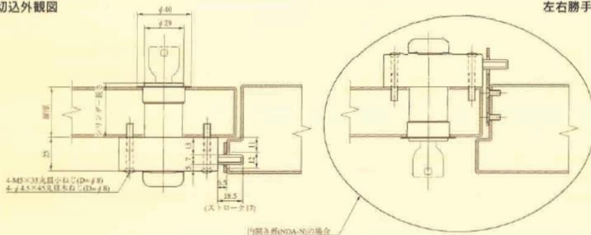
切込外観図
