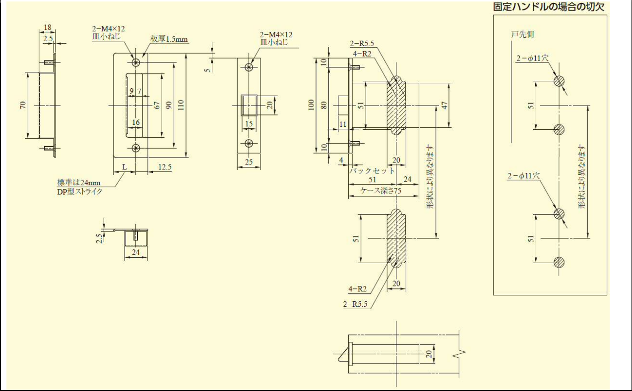
POM500シリーズの切込外観図
