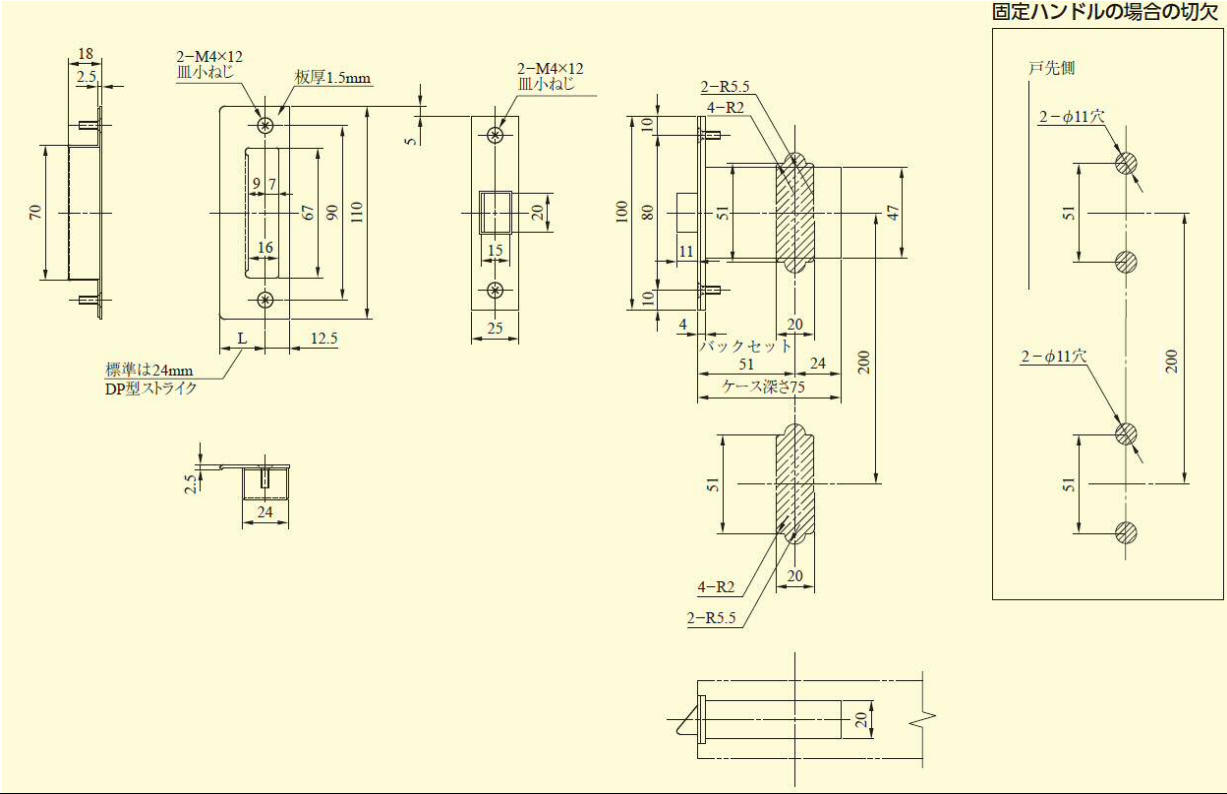
POM505、50580、506、50680の切込外観図
