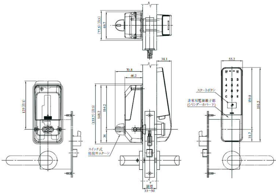
本図は TE タイプへの装着図を示します。
